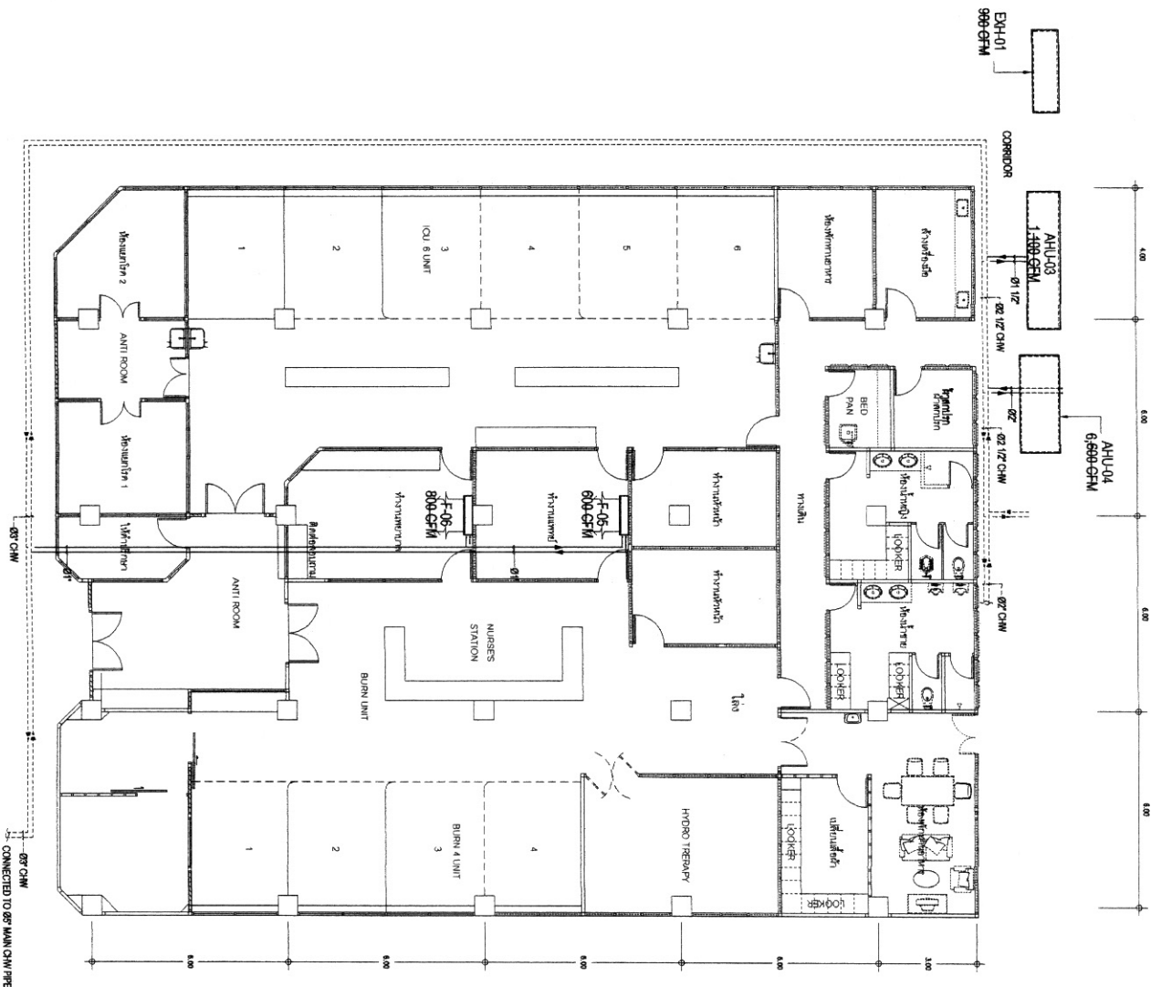
แปลนระบบปรับอากาศและระบายอากาศ ICU TM 2 มาตราส่วน 1:150
