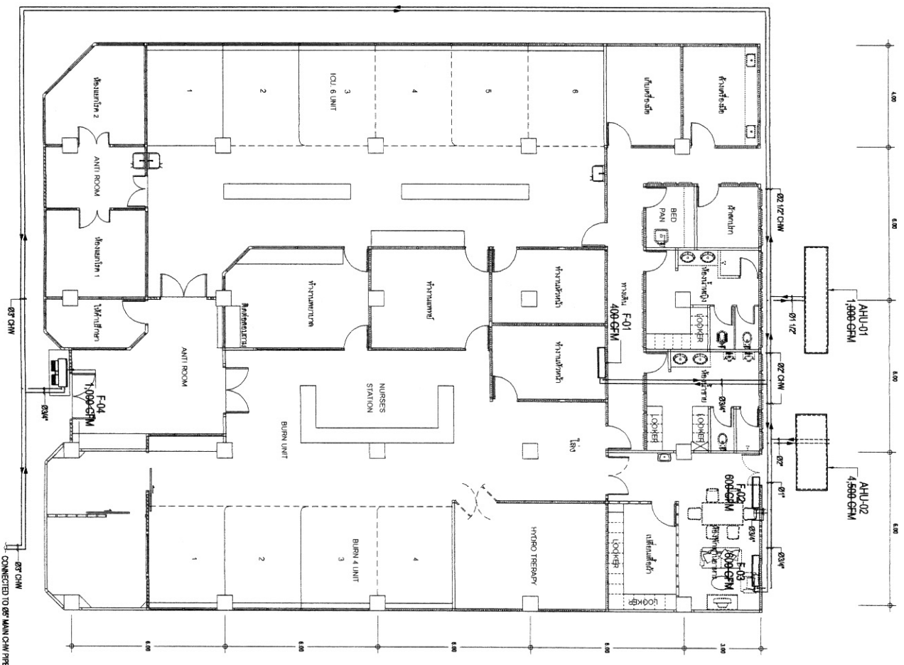
แปลระบบปรับอากาศและระบายอากาศ BURN UNIT 2 มาตราส่วน 1:150
